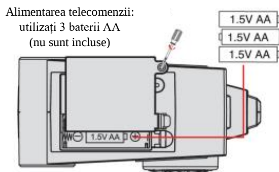
Fig.3 Instalarea bateriei de stocare pe carcasa mașinii
