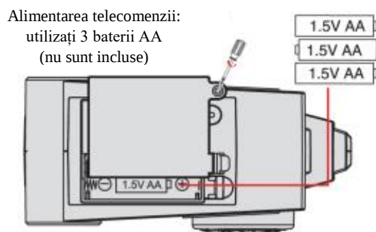
Fig.2 Instalarea bateriilor în telecomandă
