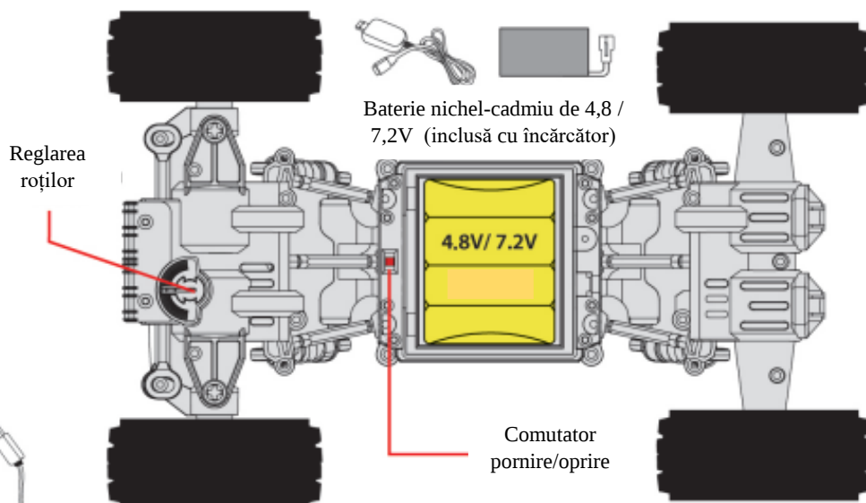
Fig.3 Instalarea bateriei de stocare pe carcasa mașinii
